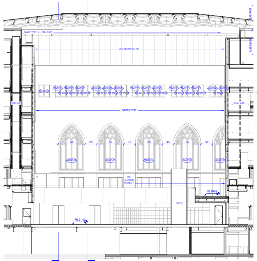
Coupe de la cour ouest, en direction ouest.
