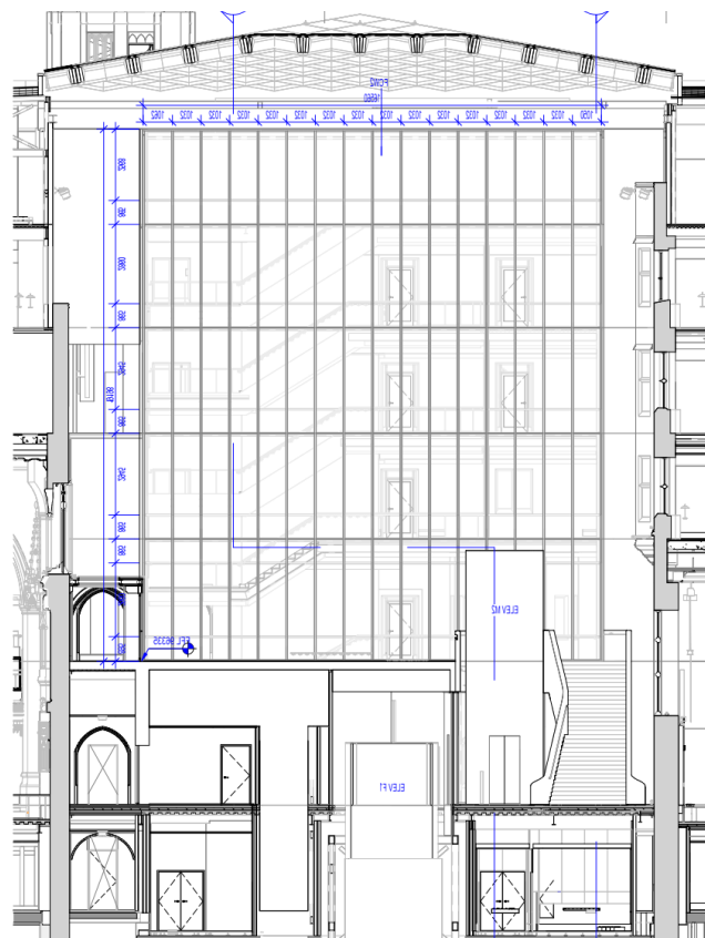
Coupe de la cour est, en direction nord.
