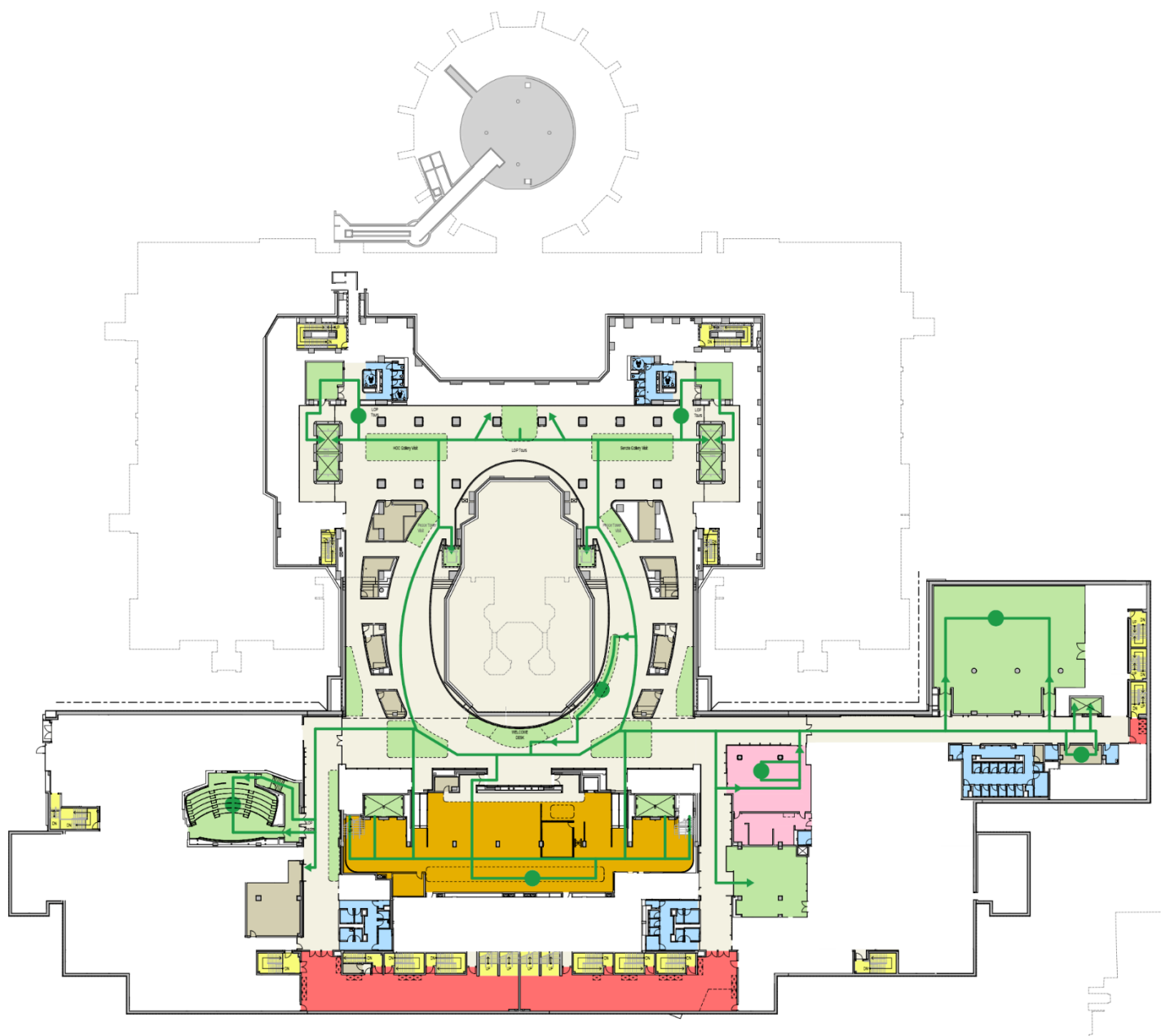
Plan de repérage du niveau B1 (sous-sol – niveau 1) du projet de Centre d'accueil du Parlement (CAP). La zone de contrôle de sécurité est indiquée en orange, les toilettes publiques en bleu clair, les espaces publics et accessibles aux visiteurs en vert clair, les aires de service en marron clair et les accès verticaux (sécurité des personnes/issues de secours) en jaune. Les parcours de circulation du public sont indiqués en vert foncé.
