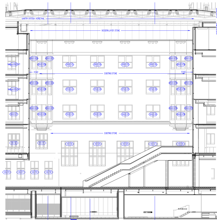
Coupe de la cour est, en direction ouest.
