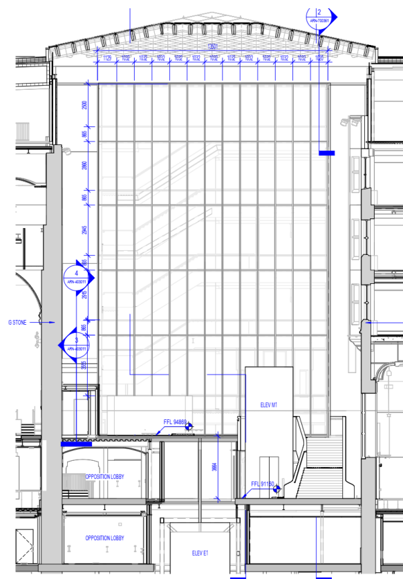
Coupe de la cour ouest, en direction nord.
