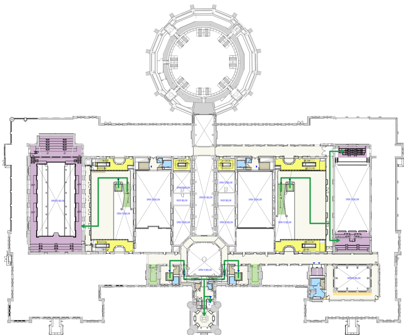
Plan de repérage du niveau 3 de l'édifice du Centre, où figurent les cours intérieures est et ouest ainsi que les tribunes de la Chambre des communes et du Sénat. Les espaces publics et accessibles aux visiteurs sont indiqués en vert clair, les tribunes de la Chambre des communes (à l'ouest) et du Sénat (à l'est) en violet, les aires de service en marron clair, et la circulation verticale (sécurité des personnes/issues de secours) en jaune. Les parcours de circulation du public sont indiqués en vert foncé.
